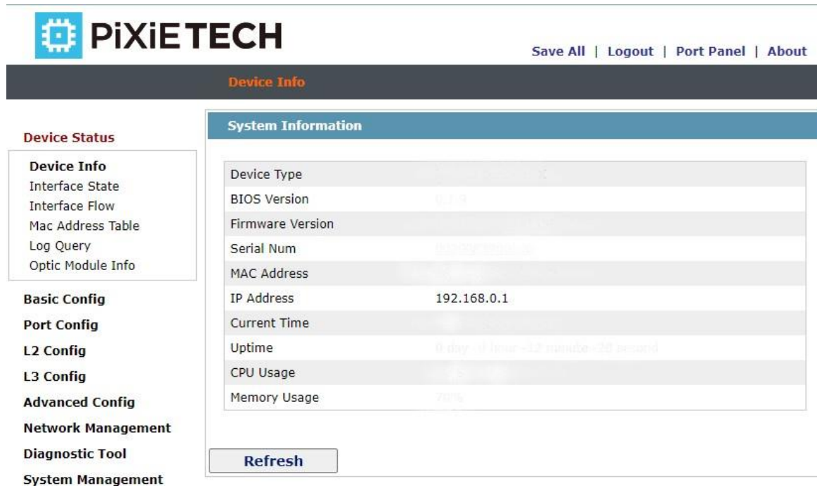
Рисунок 2: Веб-страница
